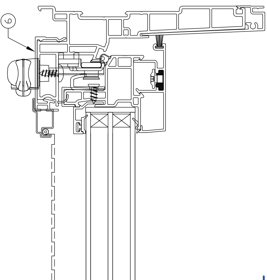
FENÊTRE À BATTANT HYBRIDE 5 3/4" 5 3/4" HYBRID CASEMENT WINDOW
